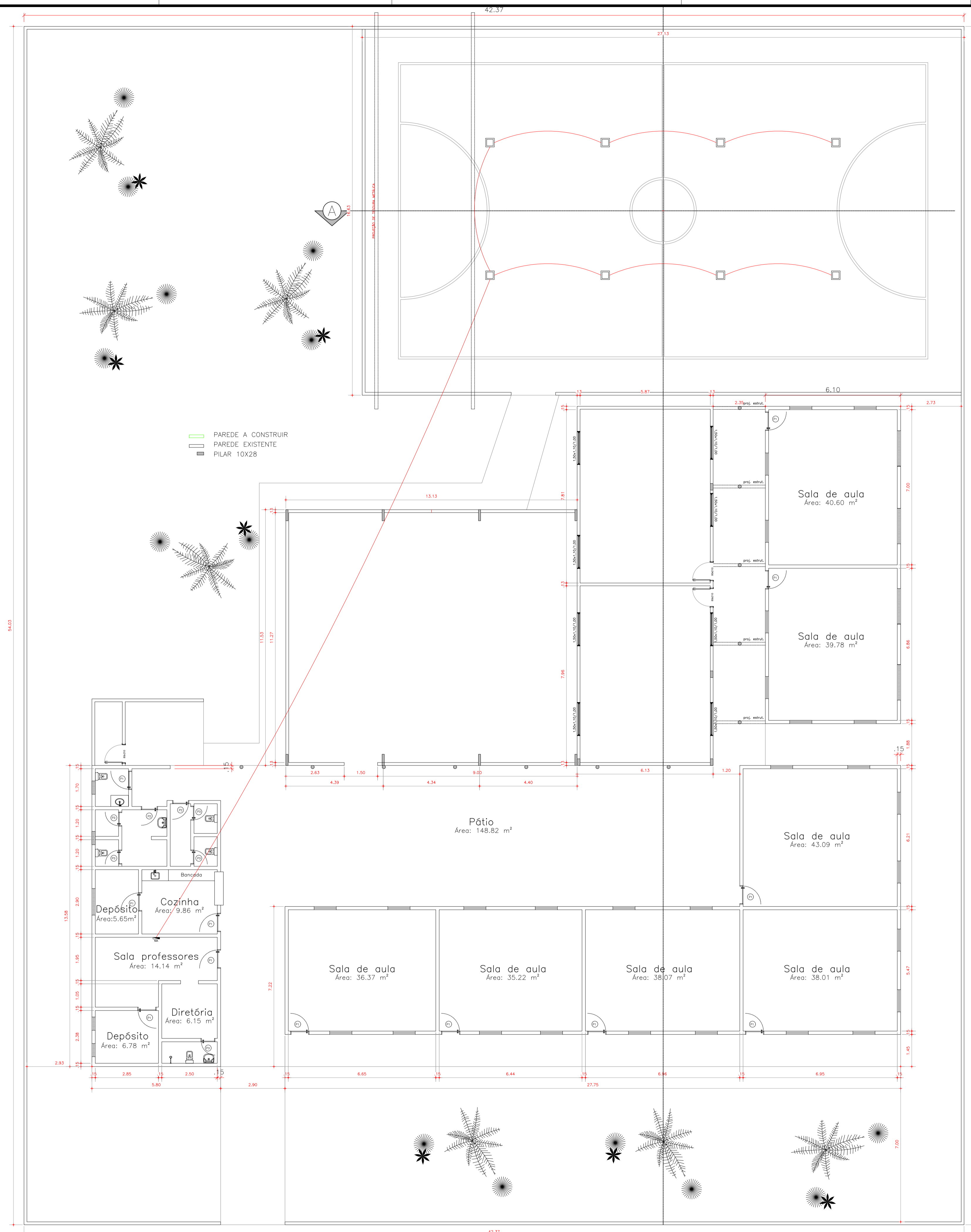
1 PLANTA BAIXA/LOC. ELÉT. ESCALA 1:100
